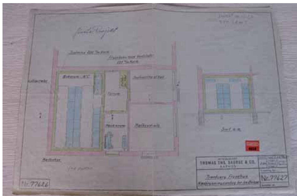
Plantegning af frysehuset
